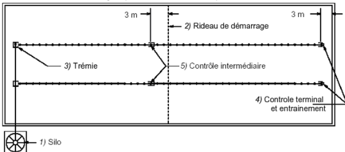
Schéma 1 : localisation des éléments pour des lignes inférieures à 120 mètres
